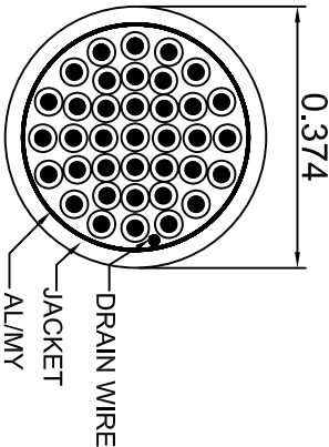
SEC A-A
