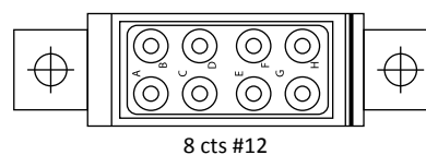
001758 401 02 A : 26,8 (1.055) B : 24,5 (.964) Masse / Weight 26 g
