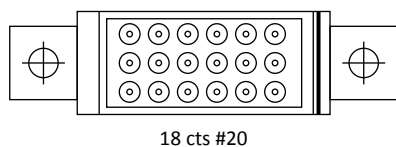
001758 201 02 sans marquage without markings A : 24,8 (.976) B : 22,5 (.885) Masse / Weight 28,0 g
