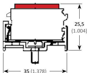
Référence Part number 001758 220 02 Masse / Weight 17,8 g
