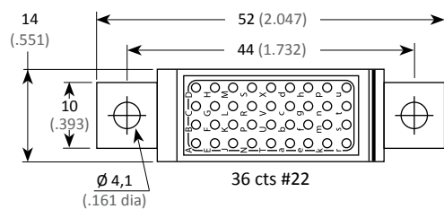
001758 101 02 A : 21,8 (.858) B : 19,5 (.767) Masse / Weight 24,0 g
