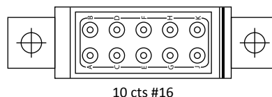
001758 301 02 A : 26,8 (1.055) B : 24,5 (.964) Masse / Weight 25 g
