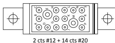
001758 501 02 A : 26,8 (1.055) B : 24,5 (.964) Masse / Weight 34 g
