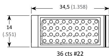
Référence Part number 001758 120 02 Masse / Weight 17,8 g
