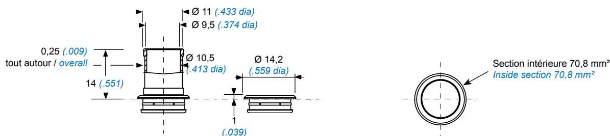
Cheminée cylindrique / Cylindrical chimney
