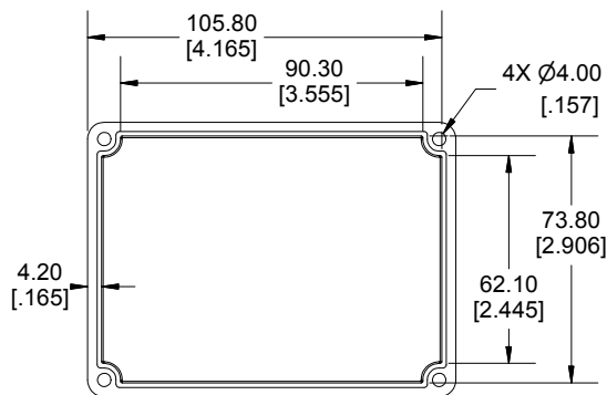
INSIDE LID
