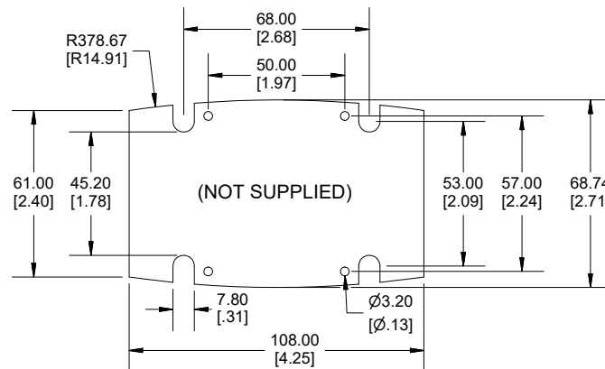
MAXIMUM P.C.B. SIZE
