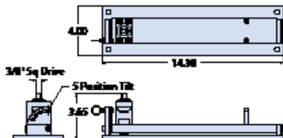
Bench Stand 600-162
