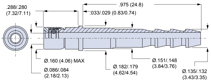
830-004 Socket Contact
