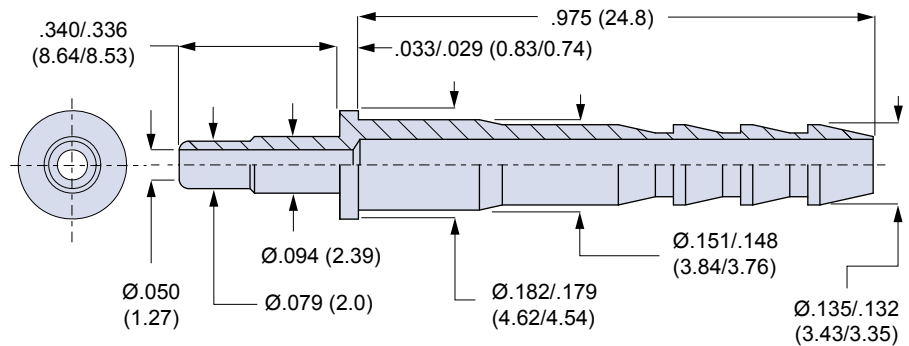
830-003 Pin Contact
