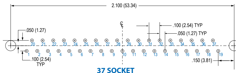
37 SOCKET
