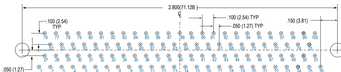
100 SOCKET
