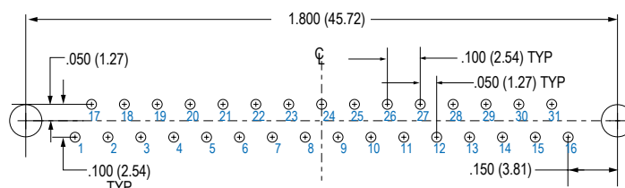
31 SOCKET
