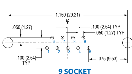
9 SOCKET
