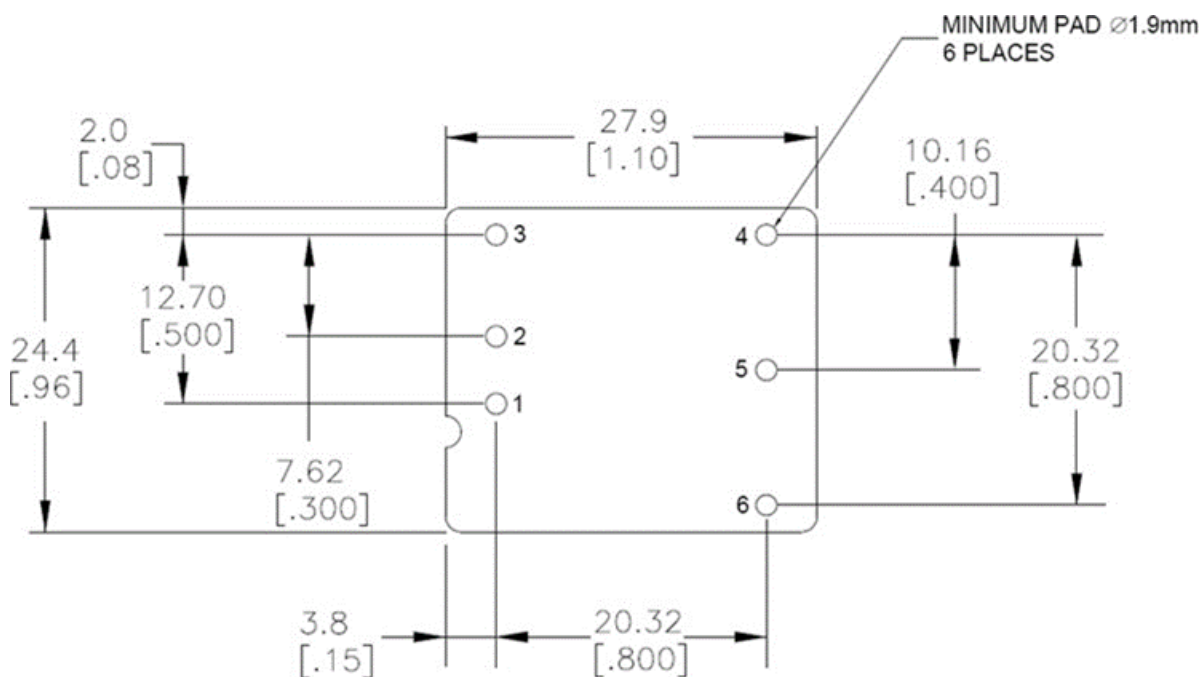
SMT Layout
