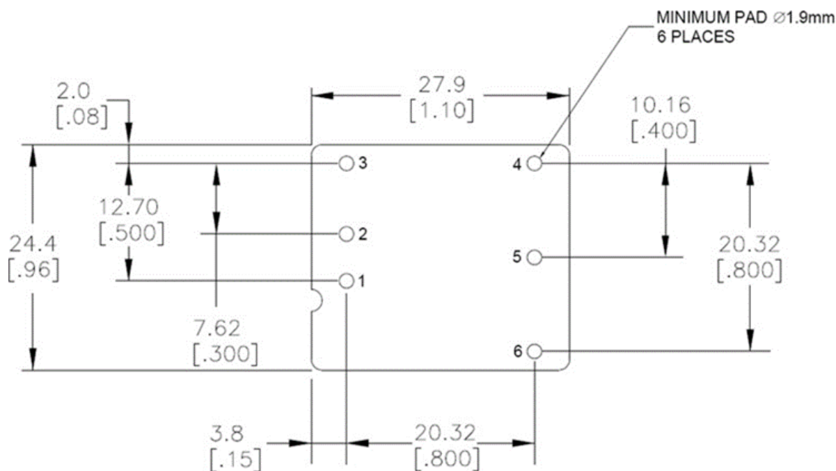
SMT Layout
