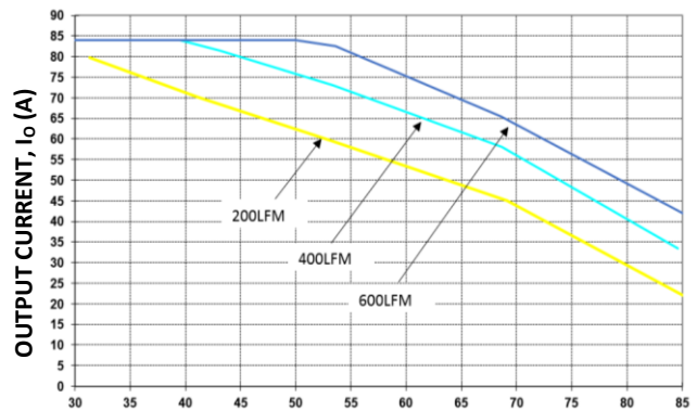
LOCAL AMBIENT TEMPERATURE, T_A (°C)
