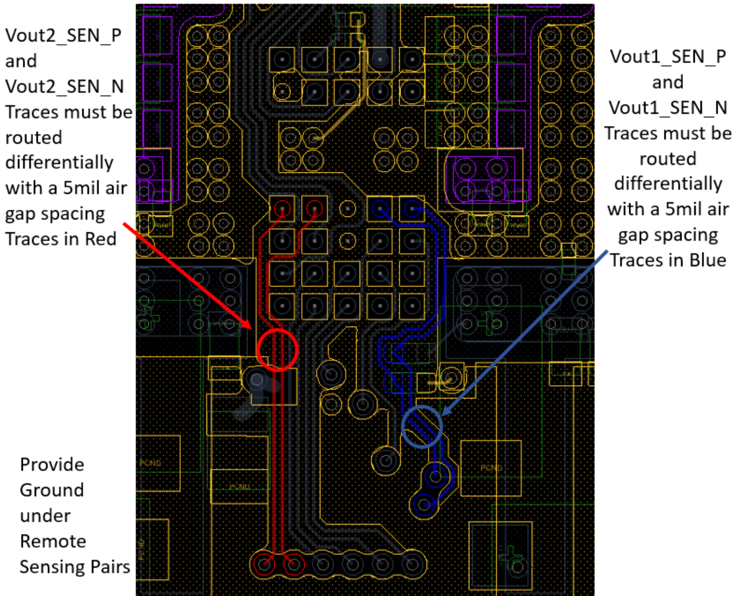
Figure 33 : VSense Traces
