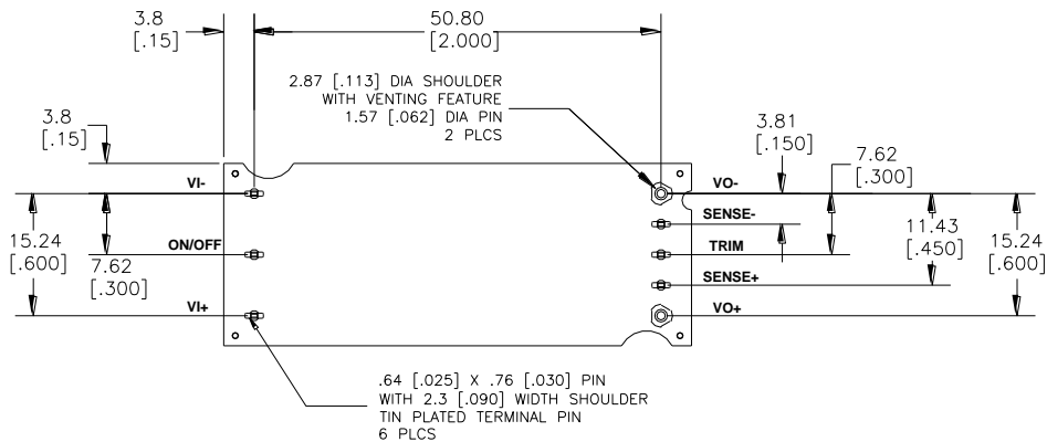
Bottom View*
