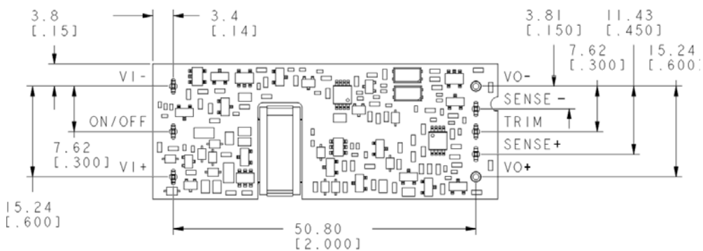
Pin Function 1 VI(+) 2 On/Off 3 VI(-) 4 Vo(-) 5 Sense(-) 6 Trim 7 Sense(+) 8 Vo(+)
