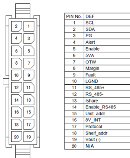
Pins Table
