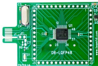
DB-LQFP48-LPC2103
