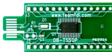
DB-TSSOP-LPC922
