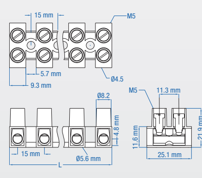
HE16 DIMENSIONS
