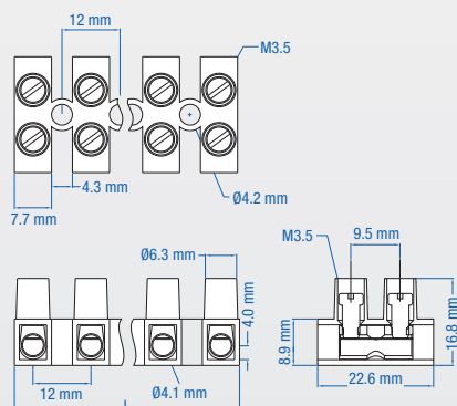
HE6 DIMENSIONS
