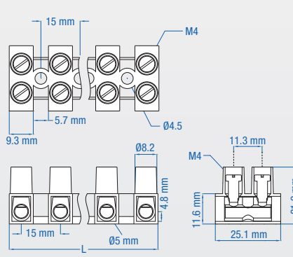
HE10 DIMENSIONS
