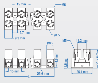
HE16 DIMENSIONS
