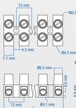
HE6 DIMENSIONS
