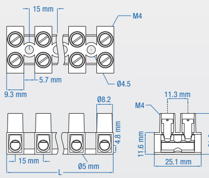
HE10 DIMENSIONS
