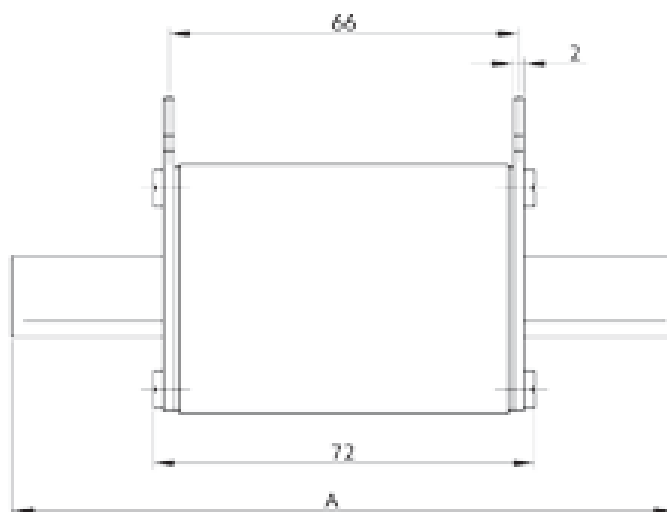
gPV, PV(gR) 750V, 1000V dimensions
