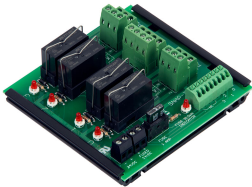
SNAP-TEX-MR10-4
