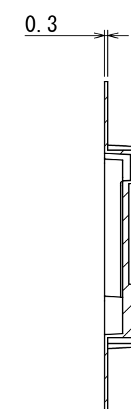
SECT B-B SCALE 2:1
