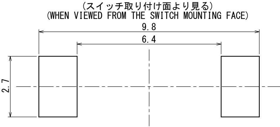
PRINTED CIRCUIT BOARD MOUNTING PATTERN DIMENSION プリント基板取り付け寸法図 (10:1)
