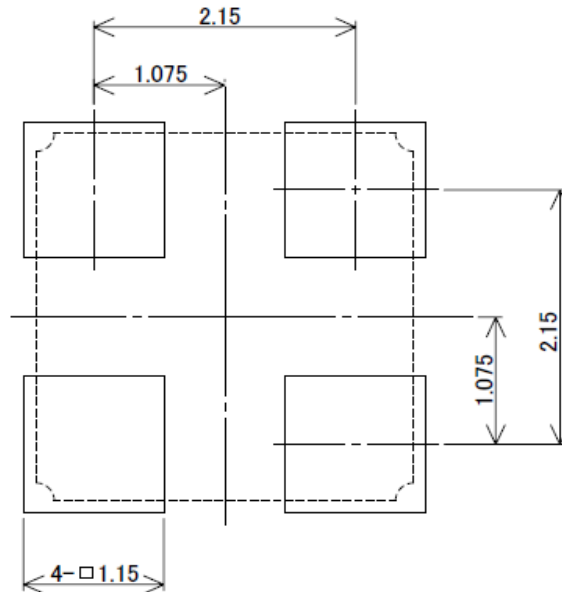
Fig. 16 : Land Pattern
