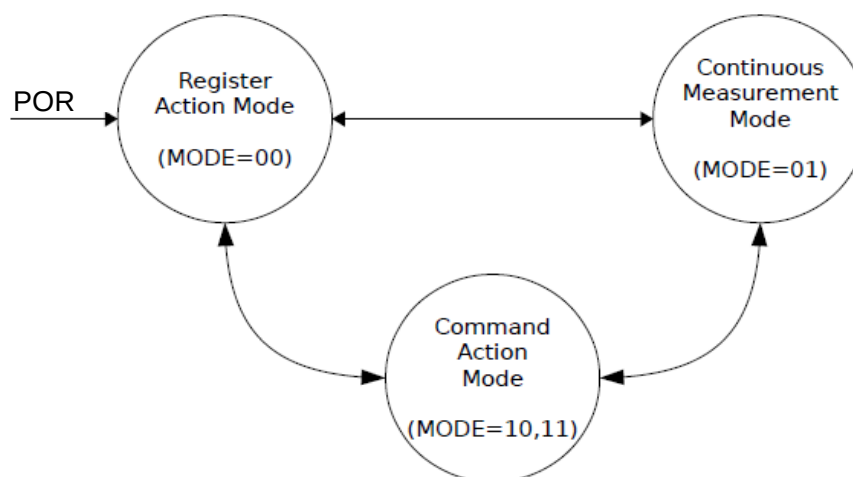
Fig. 3 : Mode transition
