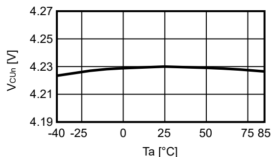
2.1 V_{CUH} vs. T_a
