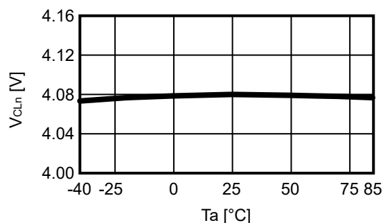
2.2 V_{CLN} vs. T_a
