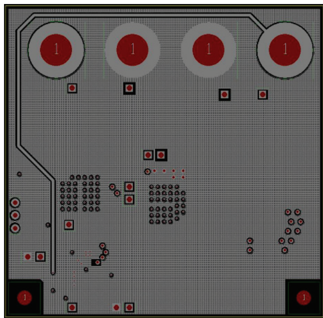
Fig. 5: Layer 2
