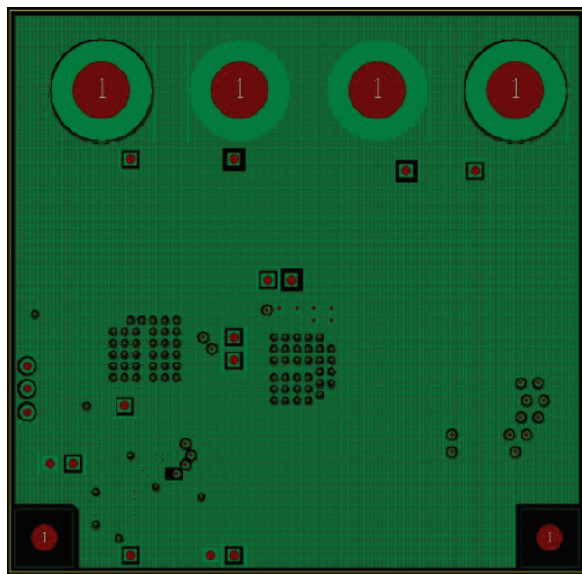
Fig. 6: Layer 3
