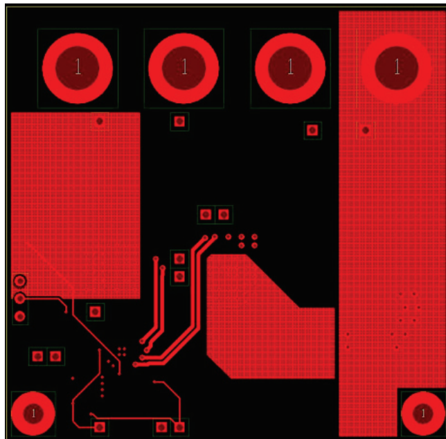
Fig. 4: Bottom Side
