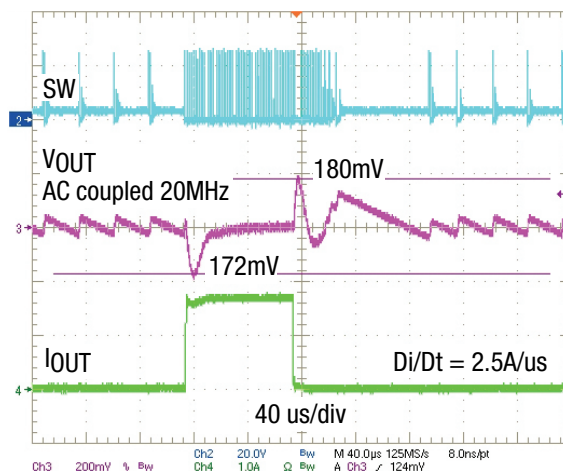
Figure 19. Load Step, DCM/CCM, 0.05\text{A}-1.5\text{A}-0.05\text{A}
