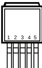
TO-263-5 Package (T5)
