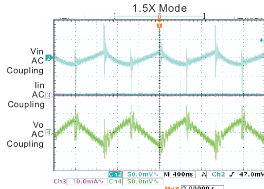
13. Output Ripple
