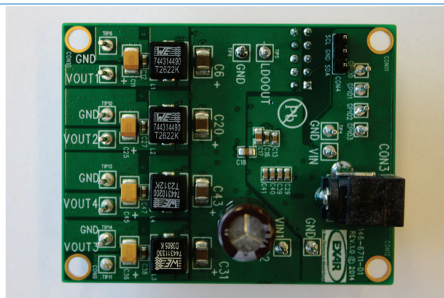
XRP7714EVB-DEMO-3
