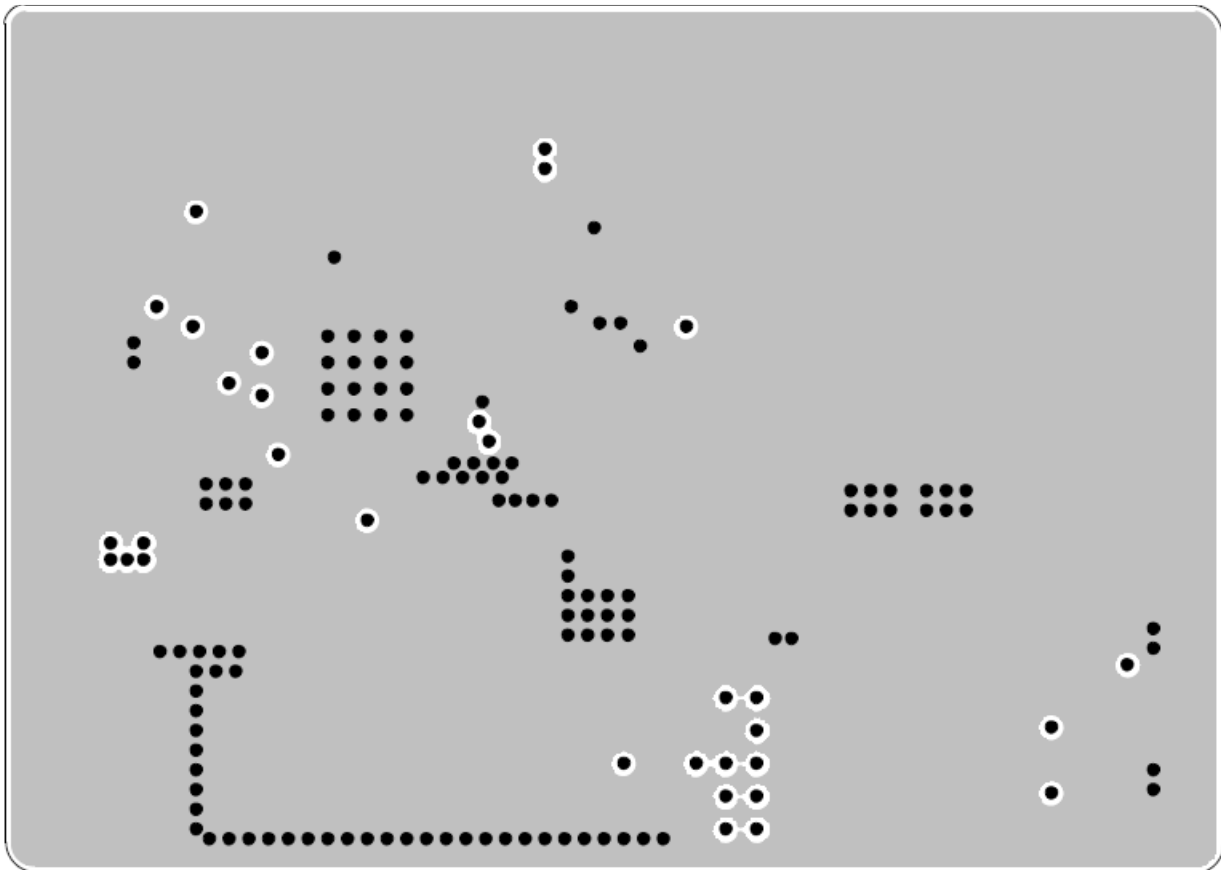
2 Inner Layer
