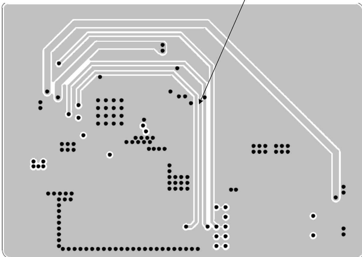
3 Inner Layer
