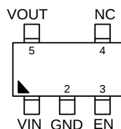
SOT-23-5
