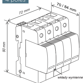
4 poles
