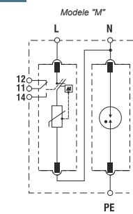
C 1+1 (2PG)
