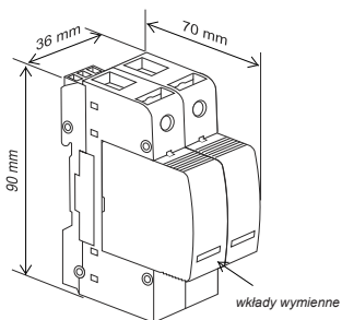
2 poles
