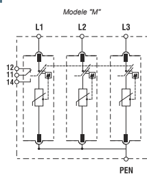
E 3+0 (3P)
