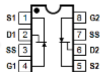
SOIC-A 8L Top View
