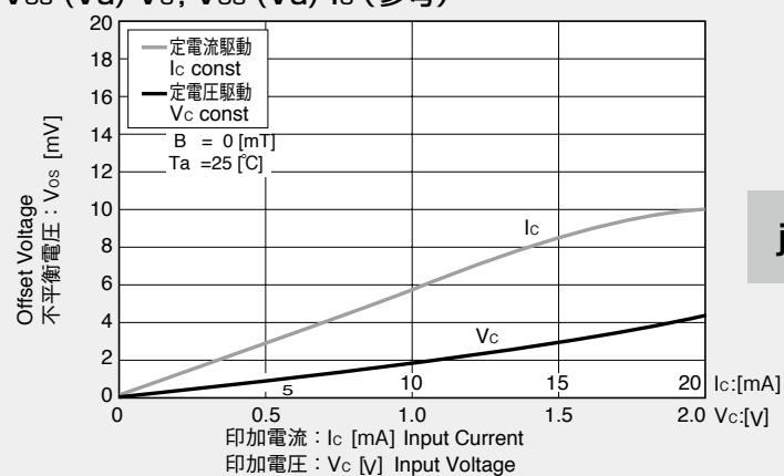
V_{os} ( V_u )- V_c , V_{os} ( V_u )- I_c (参考)
