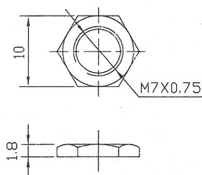
NUT 1 PC
