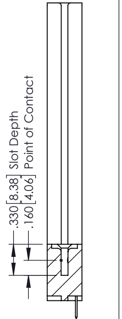
SECTION A-A
