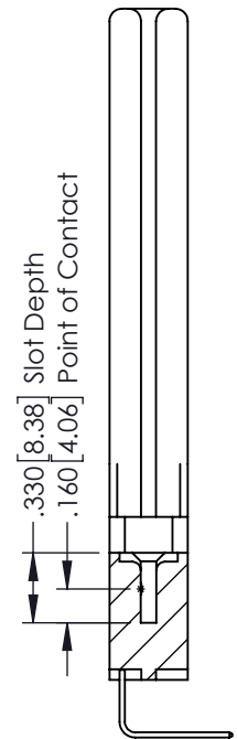
SECTION A-A
