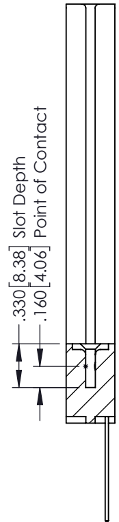
SECTION A-A
