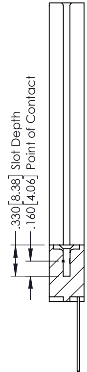
SECTION A-A
