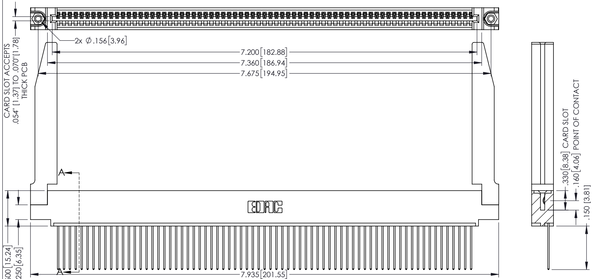
SECTION A-A
