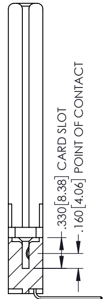
SECTION A-A
