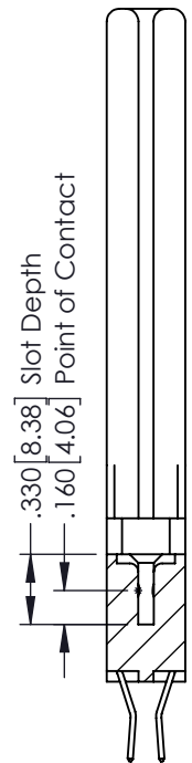
SECTION A-A
