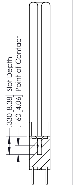
SECTION A-A
