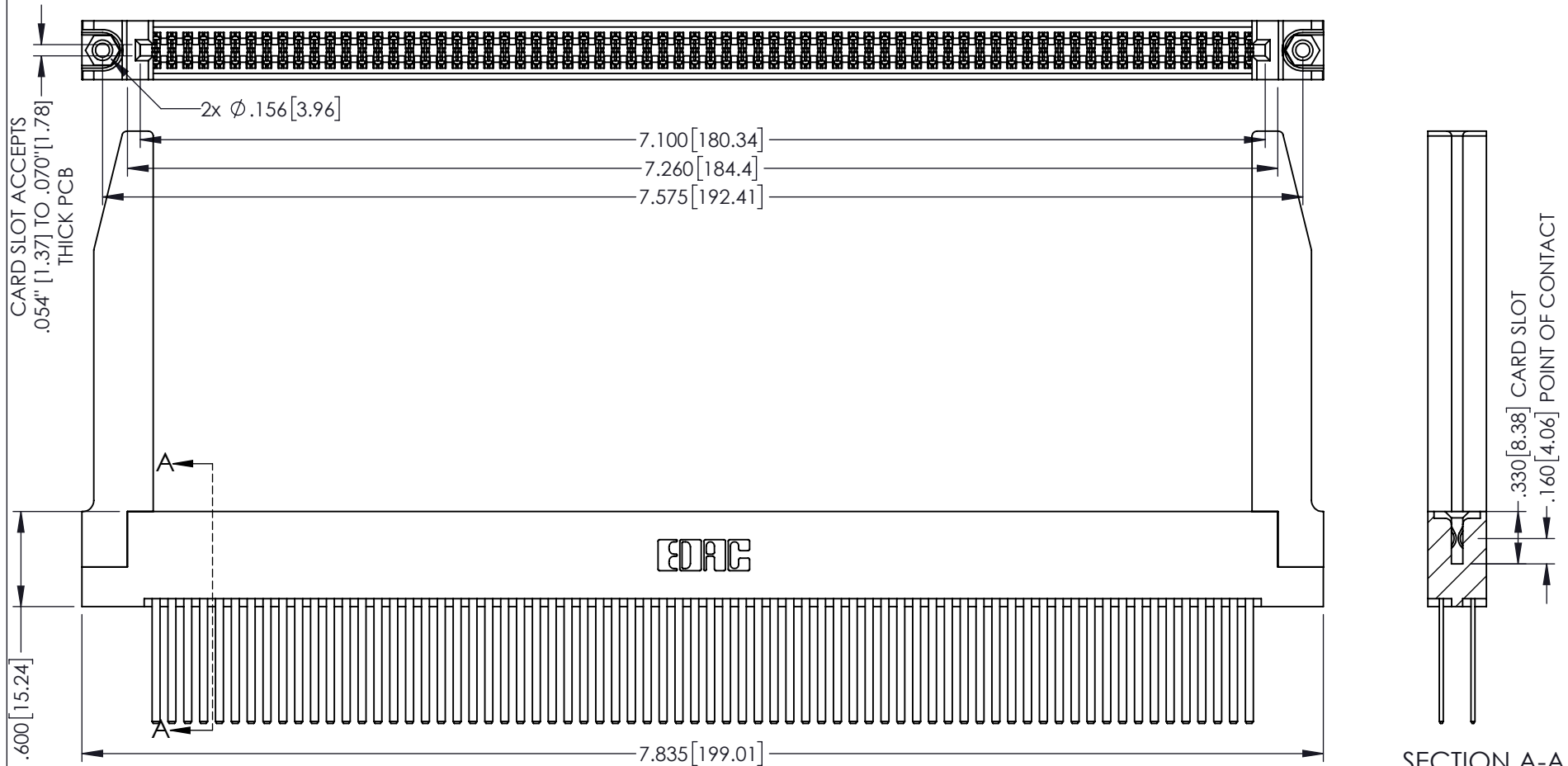
SECTION A-A
