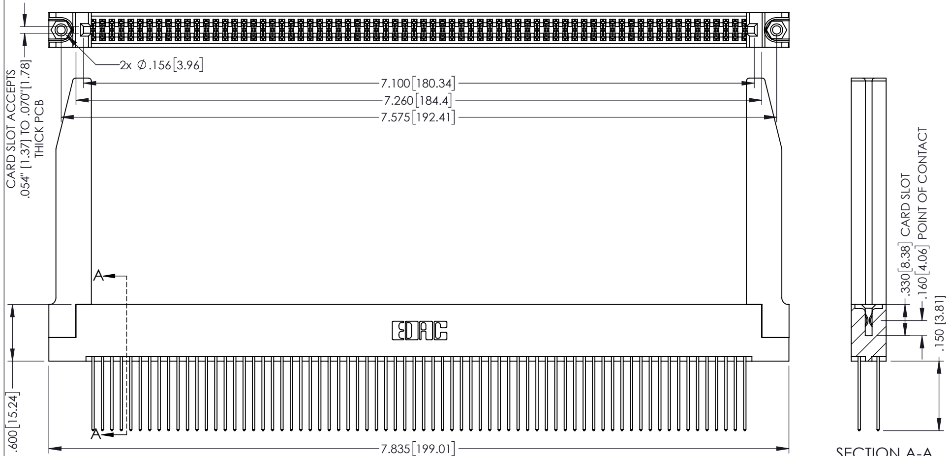
SECTION A-A
