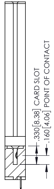
SECTION A-A
