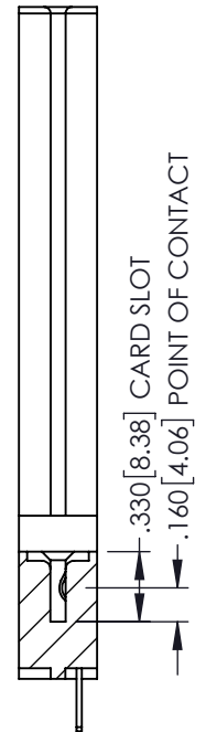
SECTION A-A
