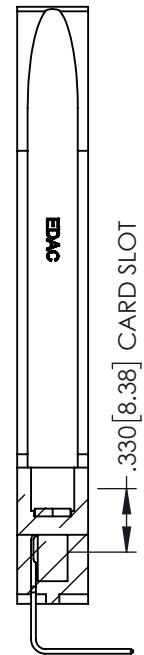
SECTION A-A
