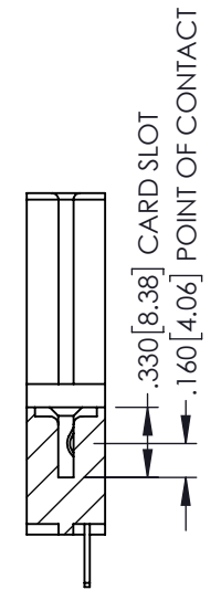
SECTION A-A
